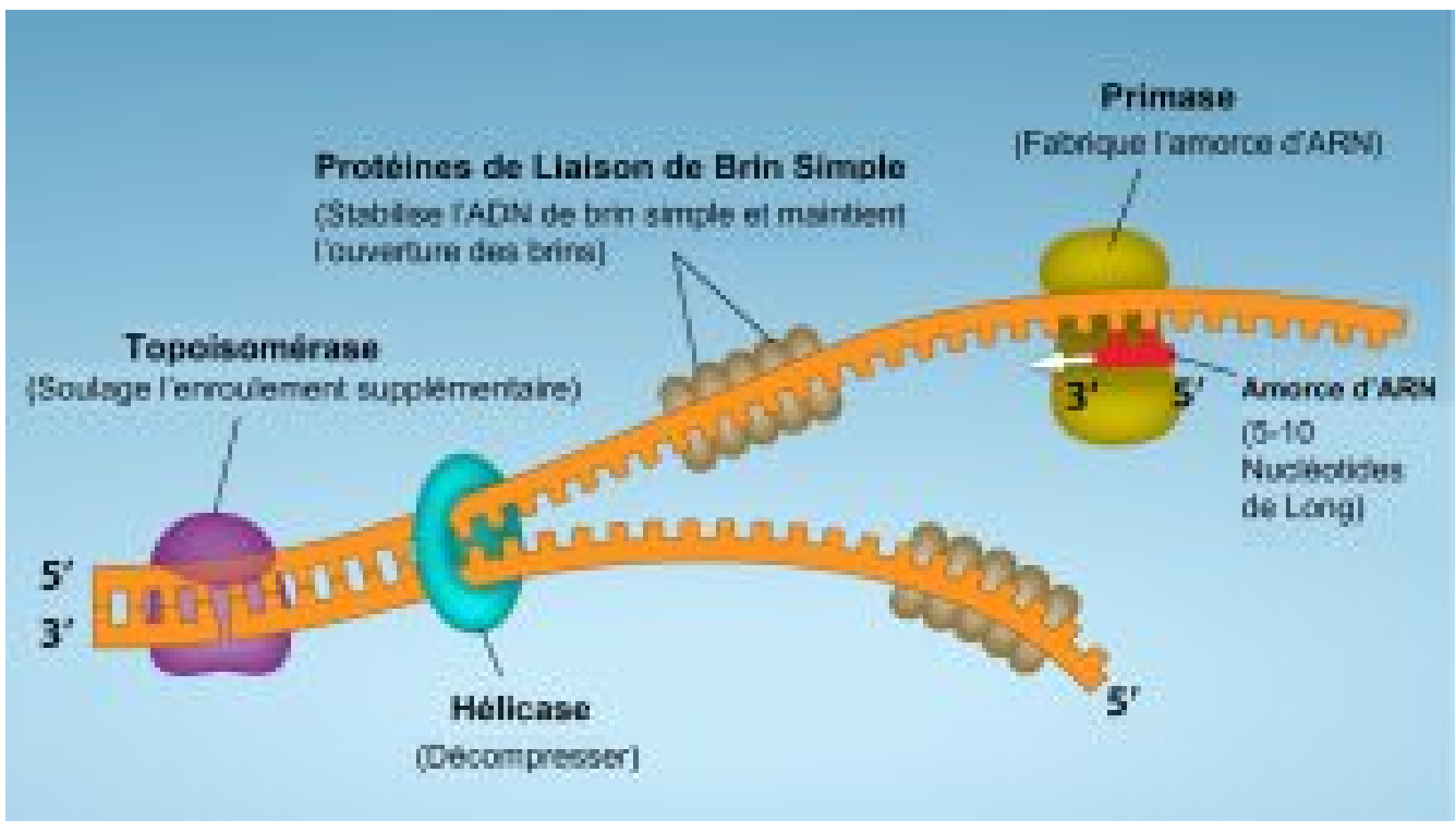
Figure 14.14 Une fourche de réplcation se forme lorsque l'hélicase sépare les brins d'ADN à l'origine de la réplcation. L'ADN a tendance à s'enrouler davantage en amont de la fourche de réplcation. La topoisomérase coupe et recolle un des deux brins d'ADN en amont de la fourche de réplcation, soulageant ainsi la pression résultant du superenroulement de l'ADN. Les protéines de liaison simple brin se lient à l'ADN simple brin pour empêcher la reformation de l'hélice. La primase synthétise une amorce d'ARN. L'ADN polymérase III utilise cette amorce pour synthétiser le brin nouveau d'ADN. Sur le brin continu, l'ADN est synthétisé en continu, tandis que sur le brin discontinu, l'ADN est synthétisé en courtes portions appelées fragments d'Okazaki. L'ADN polymérase I remplace l'amorce d'ARN par de l'ADN. L'ADN ligase scelle les liens phosphodiester entre les fragments d'Okazaki, réunissant les fragments en une seule molécule d'ADN.
