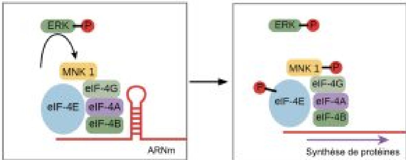
Figure 9.14. ERK est une MAP kinase qui active la traduction lorsqu'elle est phosphorylée. ERK phosphoryle MNK1, qui phosphoryle à son tour eIF-4E, un facteur d'initiation de l'élongation qui, avec d'autres facteurs d'initiation, est associé à l'ARNm. Lorsque eIF-4E est phosphorylé, l'ARNm se délie, ce qui permet à la synthèse protéique de commencer dans le noyau. (Voir la figure 9.10 pour la voie de phosphorylation qui active ERK).
