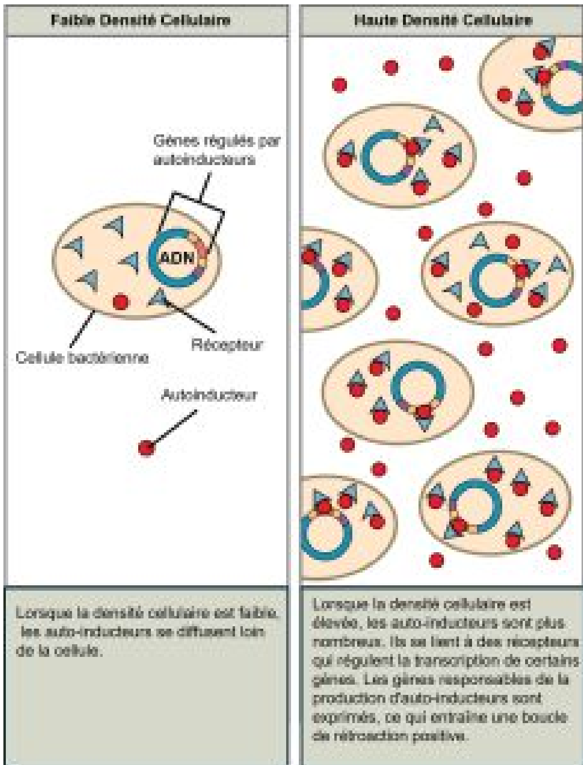
Figure 9.17. Les autoinducteurs sont de petites molécules ou protéines produites par les bactéries qui régulent l'expression des gènes.
