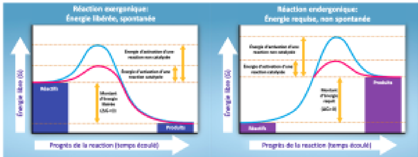
Figure 6.9 Des réactions exergoniques et endergoniques résultent dans un changement dans l'énergie libre de Gibbs ( G ). Des réactions exergoniques, en net, libèrent de l'énergie et sont des réactions spontanées. Des réactions endergoniques, en net, requièrent un investissement d'énergie pour procéder et ne sont pas des réactions spontanées. Les réactions endergoniques et exergoniques requièrent une énergie d'activation initiale pour assurer que la réaction procède. (crédit : Tag, A., Rao, A., Fletcher, S. and Ryan, A. Department of Biology, Texas A&M University)
