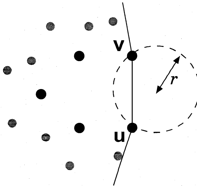
(b) Actual \alpha -shape.
