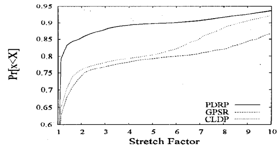
(d) 1600, d=7
