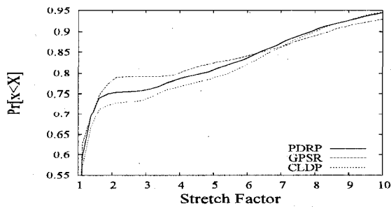
(g) 1900, d=10.4
