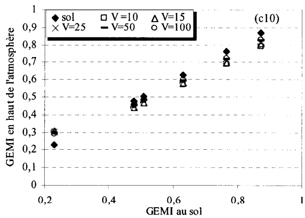
Figure 4.7 : Sensibilité des indices en fonction de la concentration en aérosols atmosphériques : (a) AVHRR, (b) VEGETATION & (c) MODIS (suite)
