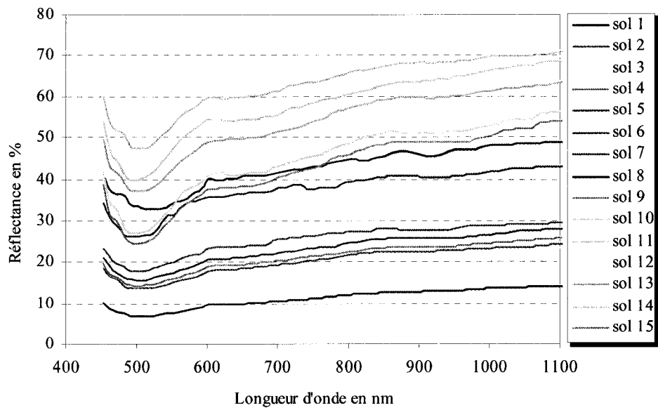
Figure 4.1 : Spectres mesurés des échantillons du premier groupe de sol nu à forte brillance
