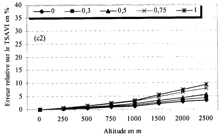
Sensibilité des indices de végétation aux effets de la topographie en fonction du taux de couverture pour une visibilité atmosphérique de 100 km pour les capteurs AVHRR(a), VEGETATION(b) et MODIS(c)
