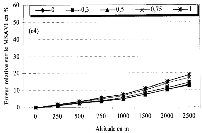
Sensibilité des indices de végétation aux effets de la topographie en fonction du taux de couverture pour une visibilité atmosphérique de 10 km pour les capteurs AVHRR(a), VEGETATION(b) et MODIS(c) (suite)
