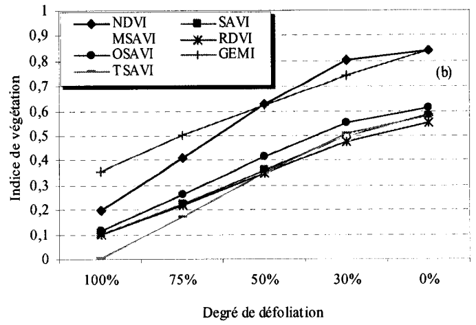
Figure 4.18 : Sensibilité des indices de végétation en fonction de la densité du couvert : cas du capteur AVHRR
