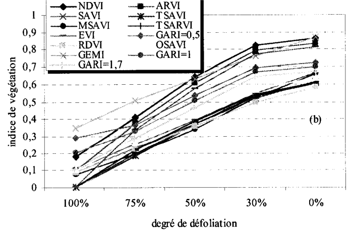
Figure 4.20 : Sensibilité des indices de végétation en fonction de la densité du couvert : cas du capteur MODIS
