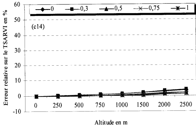
Sensibilité des indices de végétation aux effets de la topographie en fonction du taux de couverture pour une visibilité atmosphérique de 10 km pour les capteurs AVHRR(a), VEGETATION(b) et MODIS(c) (suite)
