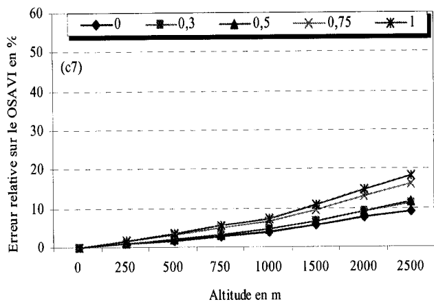
Sensibilité des indices de végétation aux effets de la topographie en fonction du taux de couverture pour une visibilité atmosphérique de 10 km pour les capteurs AVHRR(a), VEGETATION(b) et MODIS(c) (suite)
