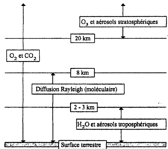
Figure 2.2 : Répartition et description des composantes atmosphériques affectant le signal dans le visible et l'infrarouge (d'après Vermote et al. , 1996)
