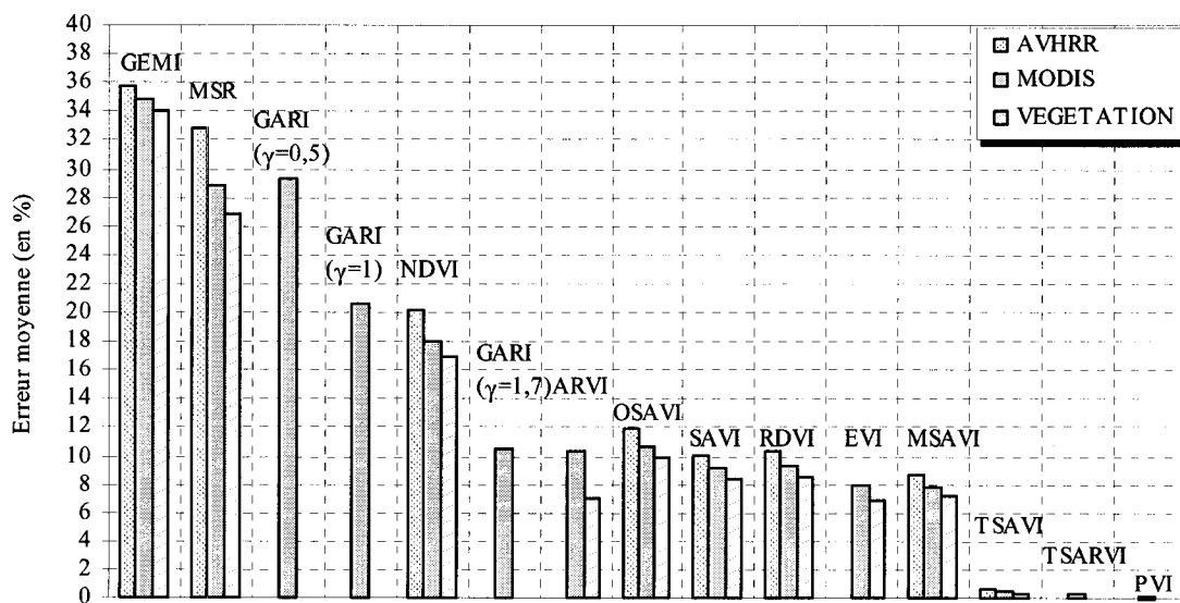
Figure 4.6 : Erreur relative moyenne de la sensibilité des indices de végétation aux propriétés optiques des sols nus en fonction des trois capteurs : AVHRR, MODIS et VEGETATION
