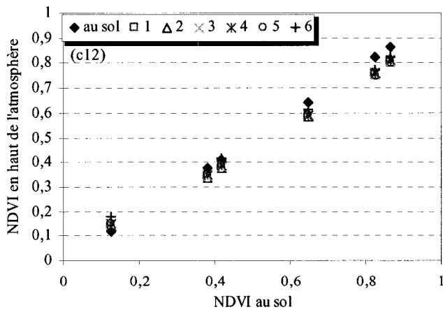
Figure 4.11 : Sensibilité des indices de végétation à l'effet de l'absorption par l'ozone : (1 :0,247g/cm 2 ); (2 :0,346g/cm 2 ); (3 :0,395g/cm 2 ); (4 :0,48g/cm 2 ); (5 :0,495g/cm 2 ); (6 :0,959g/cm 2 ) (a) AVHRR, (b) VEGETATION & (c) MODIS (suite)
