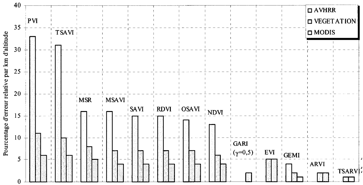
Figure 4.14 : Erreur relative moyenne de la sensibilité des indices de végétation aux effets de la topographie par km d'altitude pour une visibilité de 25 km et pour un couvert dense en fonction des capteurs AVHRR, VEGETATION & MODIS
