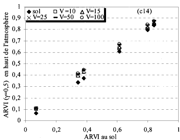
Figure 4.7 : Sensibilité des indices en fonction de la concentration en aérosols atmosphériques : (a) AVHRR, (b) VEGETATION & (c) MODIS (suite)
