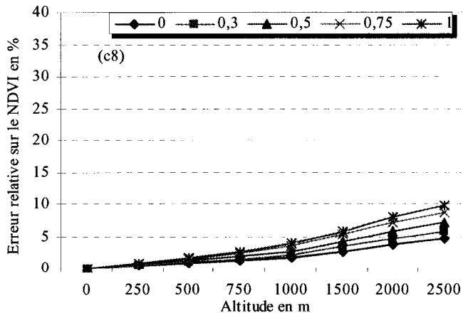
Figure 4.13 : Sensibilité des indices de végétation aux effets de la topographie en fonction du taux de couverture pour une visibilité atmosphérique de 25 km pour les capteurs (a) AVHRR, (b) VEGETATION et (c) MODIS (suite)
