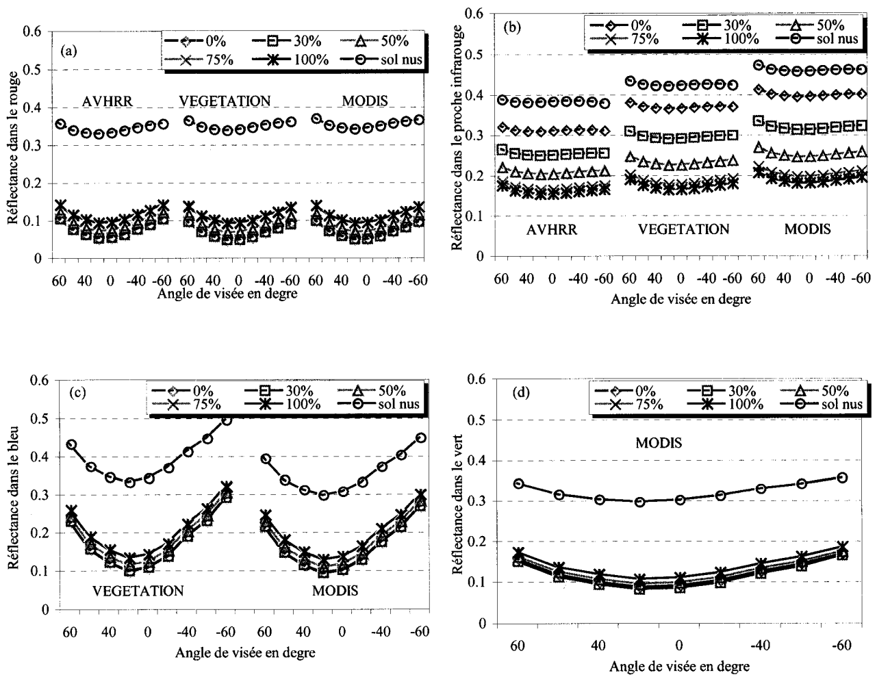
Figure 4.15 : Réponses spectrales des bandes du visible et du proche infrarouge en fonction de l'angle de visé et du capteur satellitaire
