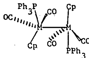
50
