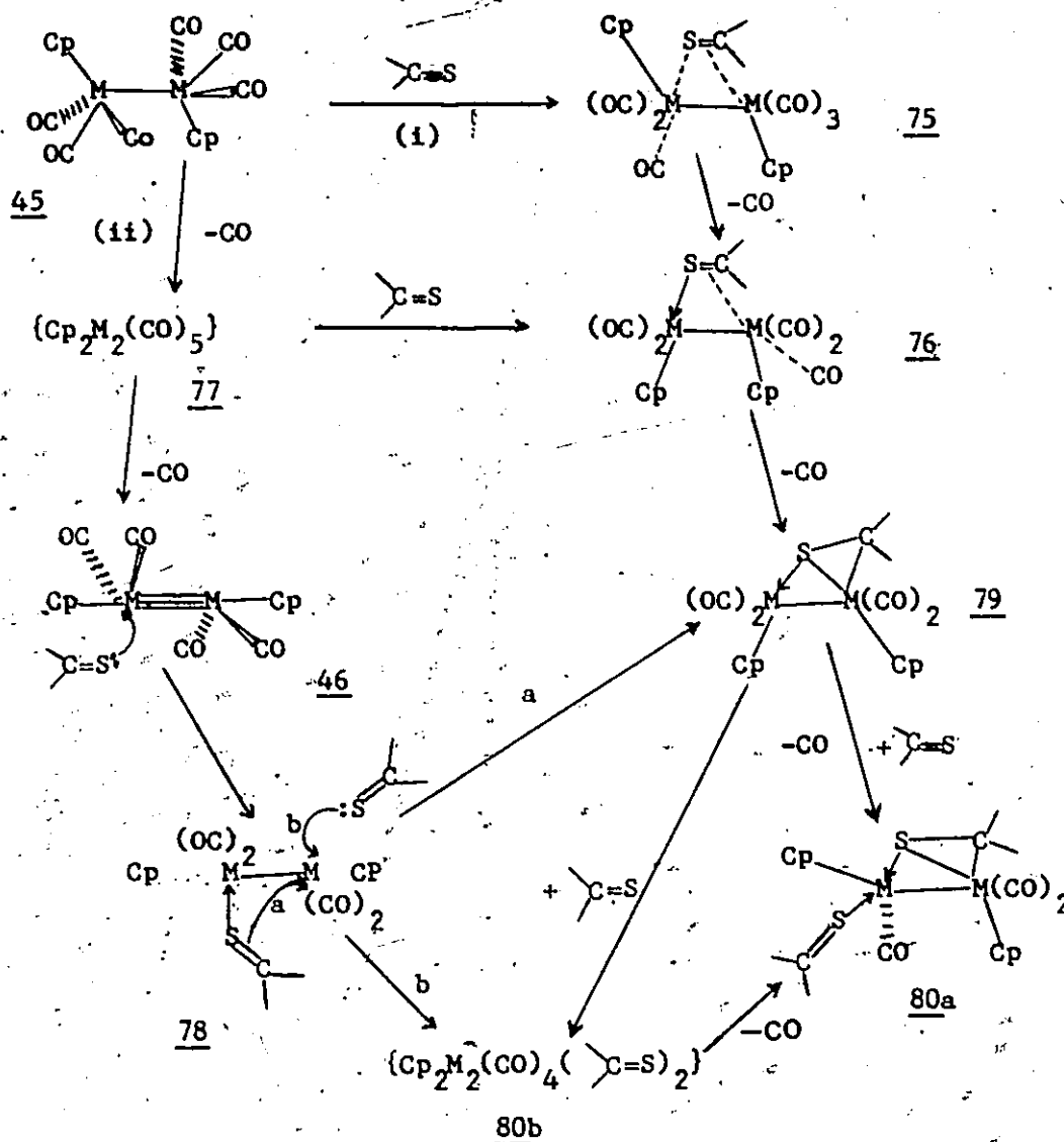
Scheme XII (M=Mo,W; \text{C=S} =thione)
