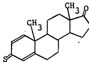
71
