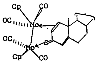
92
