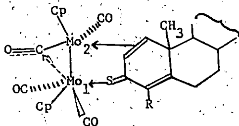
92b (R=CH 3 , H)
