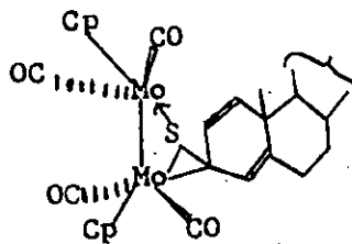
93
