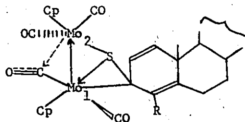
93b (R=CH 3 , H)
