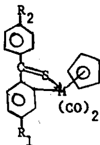
53
