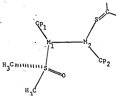
107
