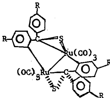
18
