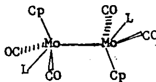
82 (L=thione)
