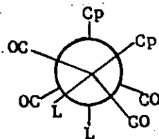
105 (b) : gauche
