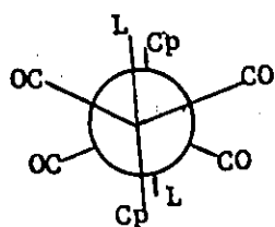
105 (a) : trans
