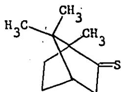
Thiocamphor ( V )
