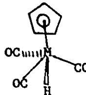
97
