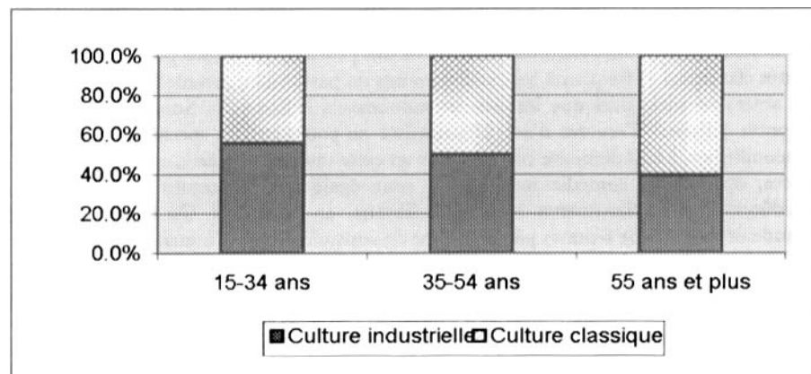
Graphique 5 - Répartition des composantes du marché de la culture en fonction de l'âge
