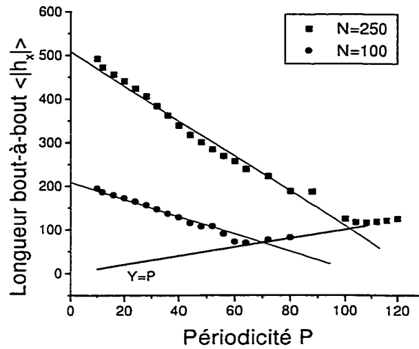
FIG. 4.9 – Longueur bout-à-bout du polymère ( \langle h_x \rangle , composante x) en fonction de la périodicité du tunnel ( P ) pour deux tailles de polymère. Le champ est \varepsilon = 0.003 .
