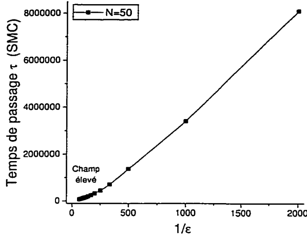
FIG. 4.27 – Temps de passage en fonction de l'inverse du champ ( \epsilon^{-1} ) pour un polymère de taille N = 50 et une profondeur de potentiel U = 1.1 .
