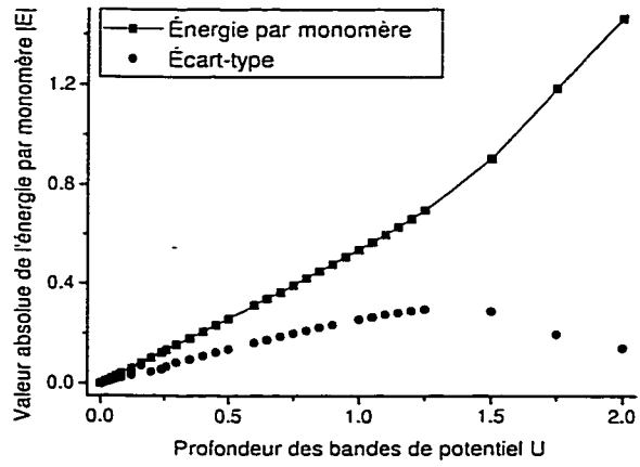
FIG. 4.33 – Valeur absolue de l'énergie par monomère normalisée (et son écart-type) en fonction de la profondeur des puits de potentiel U , pour un polymère de taille N = 100 et un champ de \varepsilon = 0.006 .
