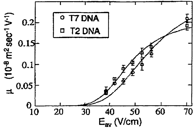
FIG. 4.25 – Mobilité en fonction du champ ( \epsilon ) pour l'ADN T2 (164 kbp) et l'ADN T7 (37.9 kbp).
